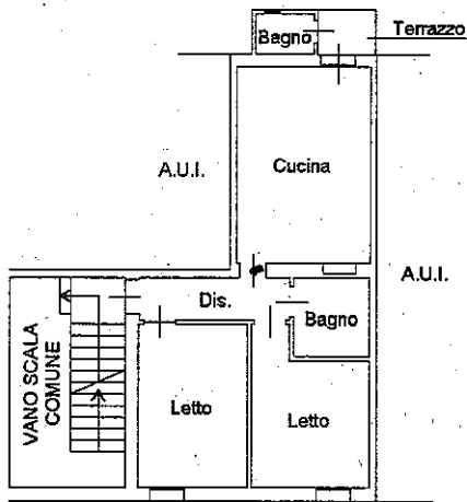
PIANO PRIMO H.3.05
